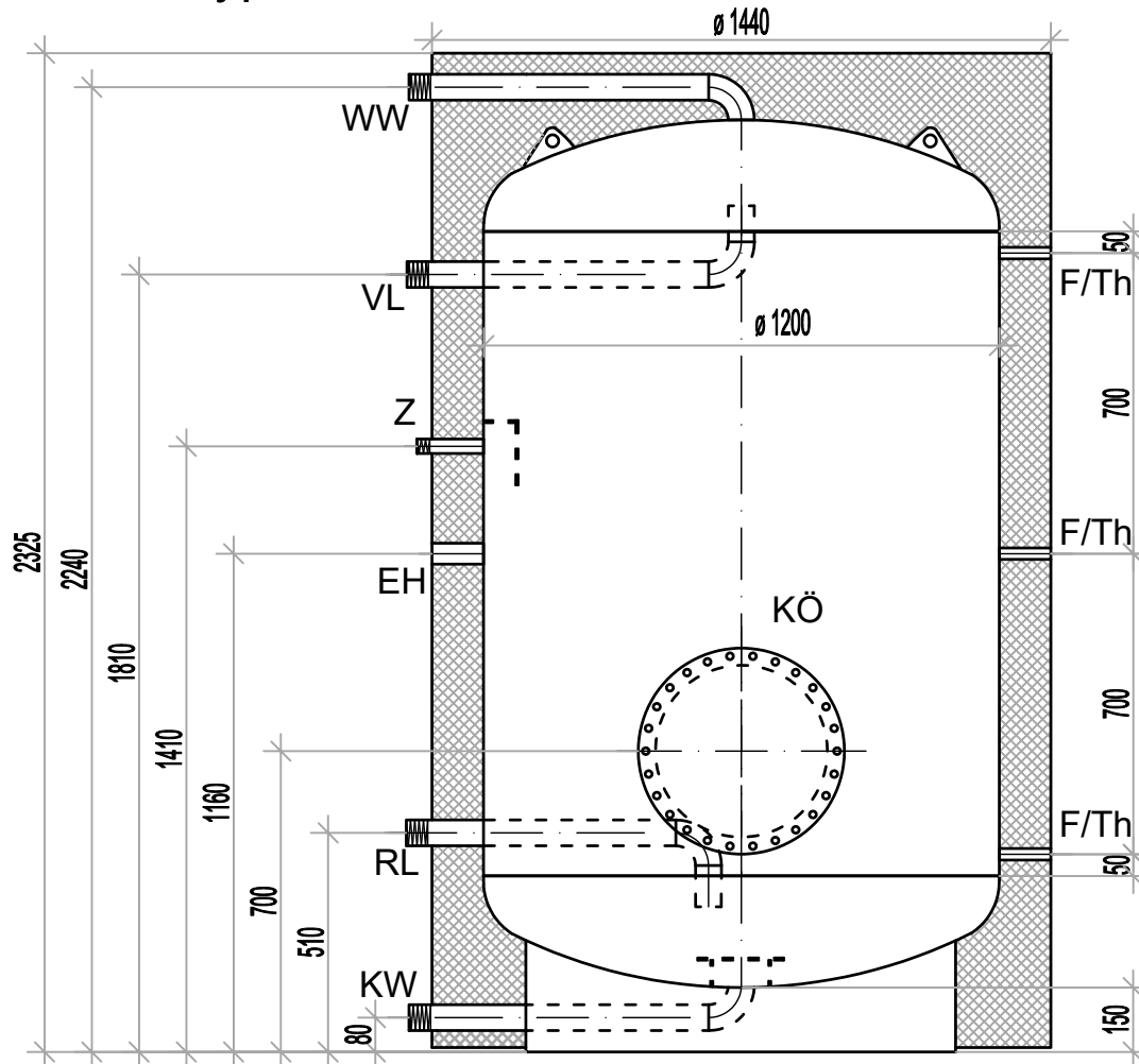
Anschlussstellung 1
